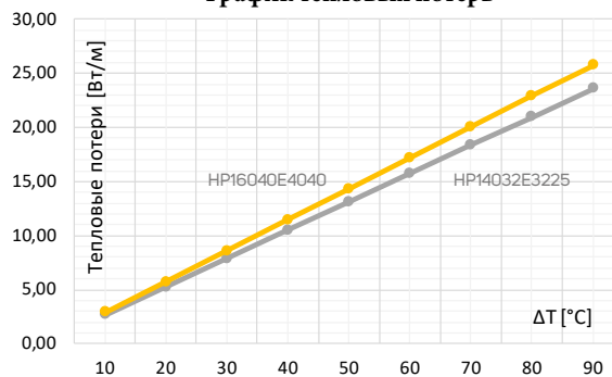
График тепловых потерь
